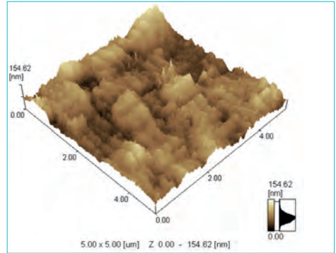
PARION AFM görüntüsü
